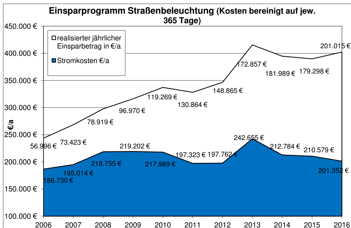
Abb. 8: Energiekosten Straßenbeleuchtung
